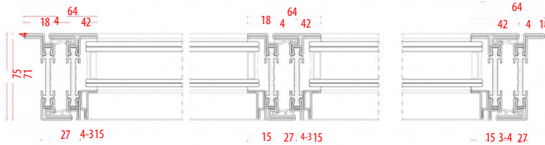
Double leaf door Inward Opening
