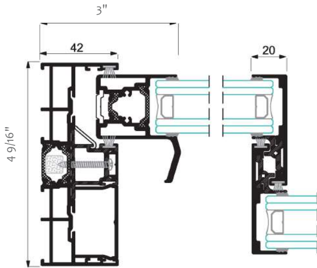
Door - cross-section KLAR VISION
