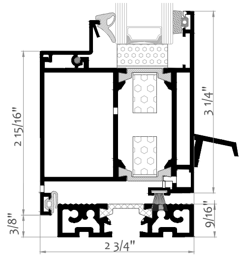
Door – cross-section KLAR-70
